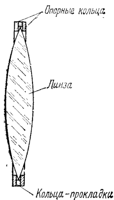
Рис. 64. Объектив трубы
