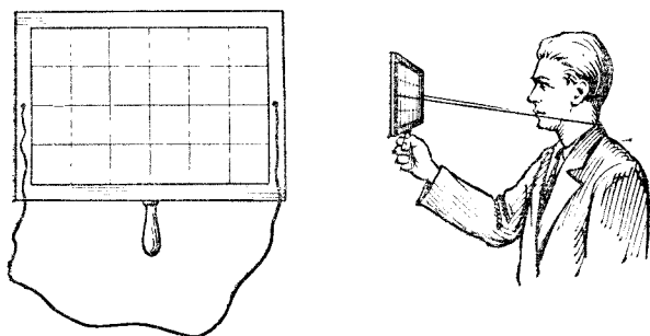
Рис. 40. Рамка для наблюдений положения планет
