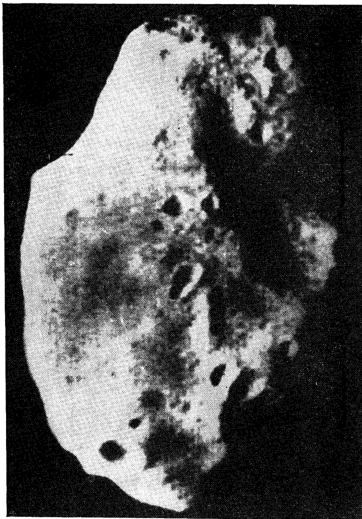
Рис. 49. Фотография Фобоса (фото «Маринера-9»)
