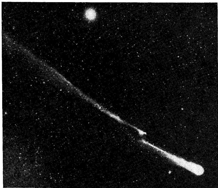
Рис. 60. Комета Галлея 10 января 1986 г. (фото получено Г. Кимеридзе, Абастуманская астрофизическая обсерватория АН Груз.ССР)
