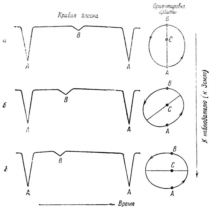
Рис. 34. Вид кривой блеска в зависимости от ориентировки орбиты звезды-спутника
