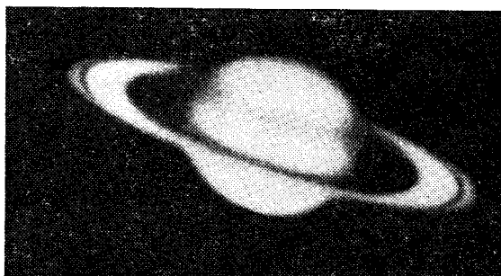
Рис. 51. Планета Сатурн
