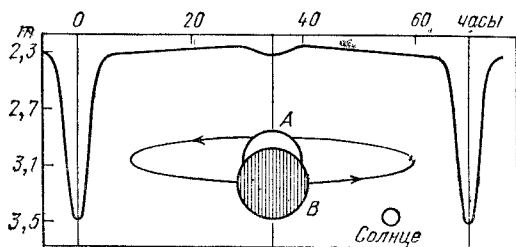
Рис. 33. Затменная переменная звезда Алголь и кривая ее блеска
