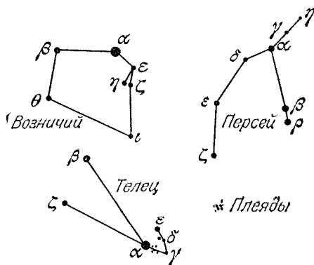
Рис. 20. Окрестности созвездия Тельца
