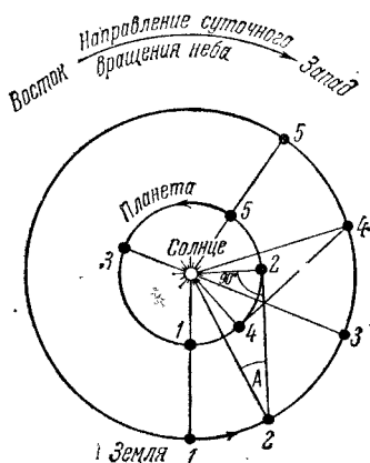
Рис. 41. Конфигурации нижних планет
