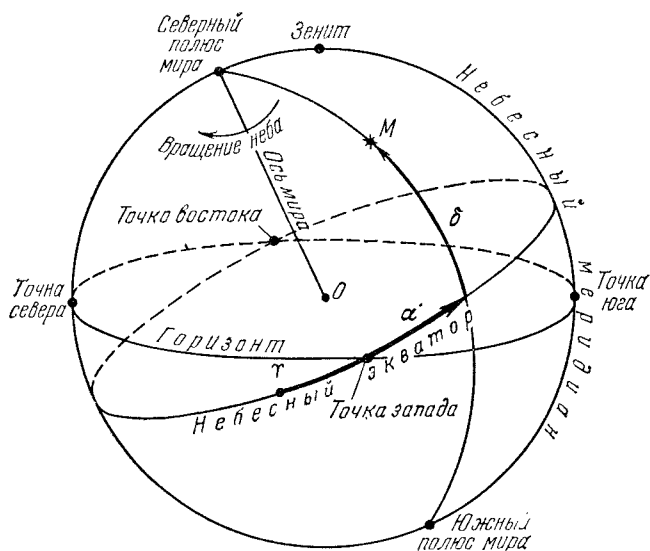
Рис. 10. Небесные экваториальные координаты. O — наблюдатель; \gamma — точка весеннего равноденствия; \alpha — прямое восхождение и \delta — склонение светила M
