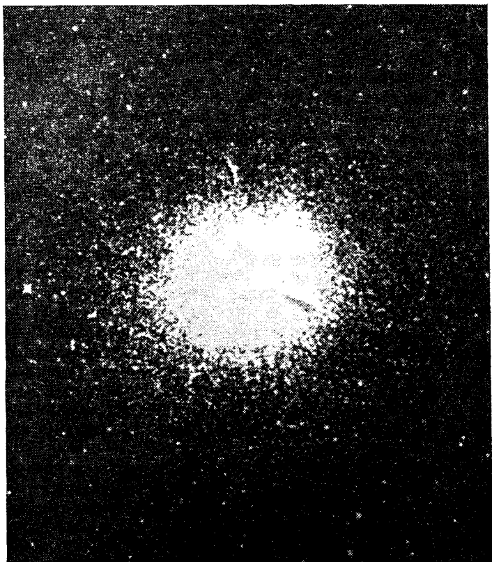
Рис. 32. Шаровое звездное скопление
