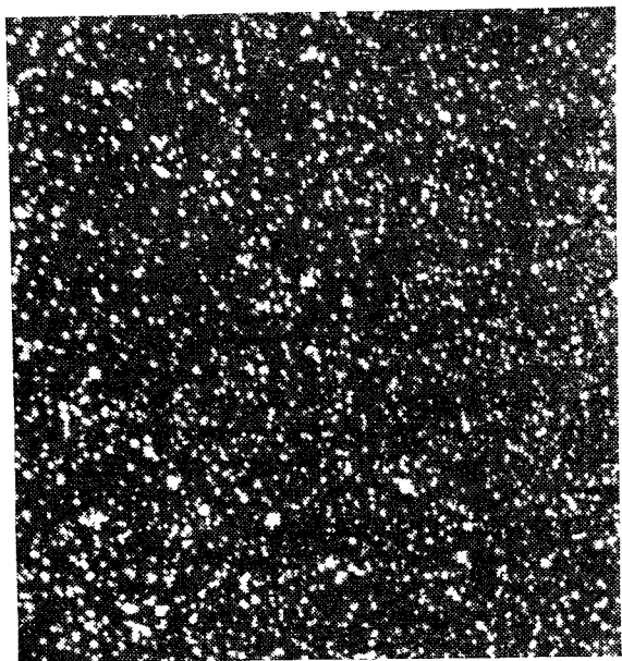
Рис. 26. Млечный Путь в созвездии Лебеда
