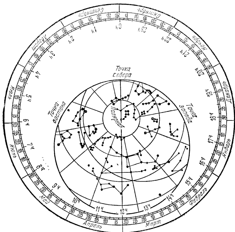
Рис. 22. Подвижная карта звездного неба
