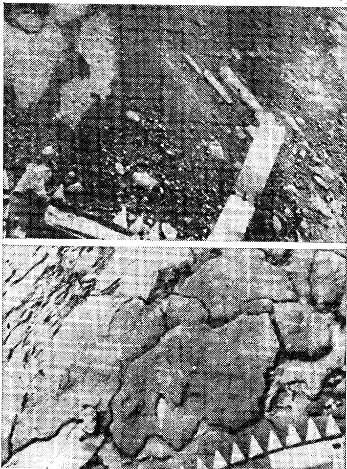
Рис. 46. Поверхность Венеры в местах посадки спускаемых аппаратов «Венера-13» (вверху) и «Венера-14» (внизу)
