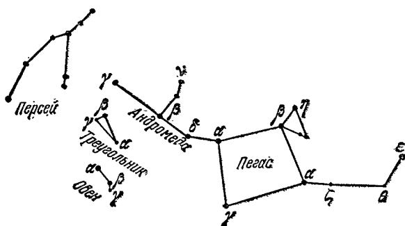
Рис. 19. Окрестности созвездия Пегаса
