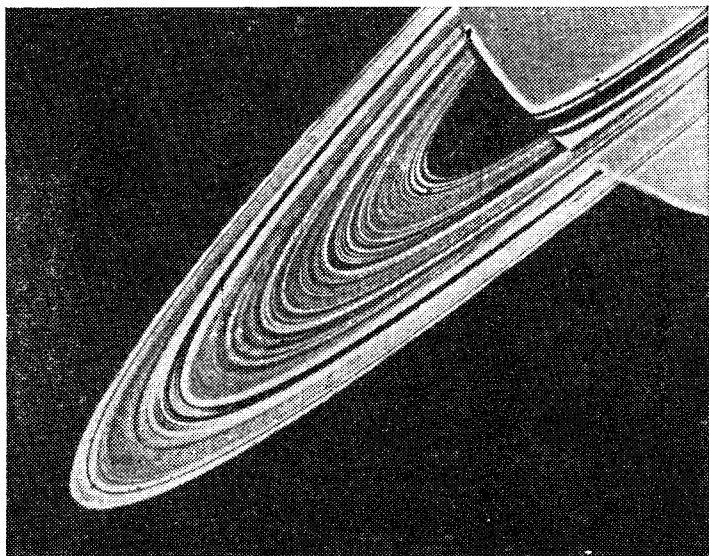
Рис. 52. Тонкая структура колец Сатурна (фото «Вояджера-1»)
