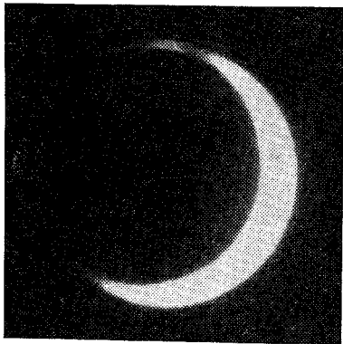
Рис. 44. Рога Венеры
