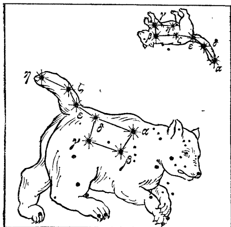
Рис. 1. Созвездия Большой и Малой Медведицы
