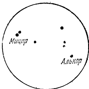
Рис. 29. Мицар и Алькор в поле зрения телескопа
