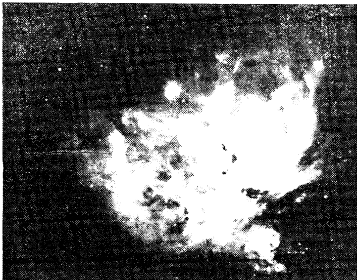
Рис. 37. Большая диффузная туманность в Созвездии Ориона
