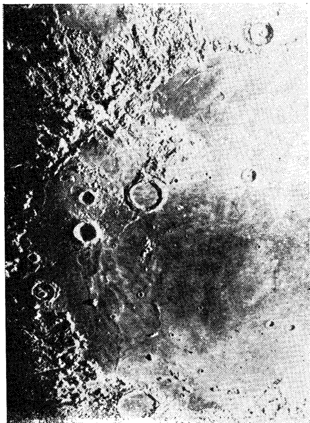
Рис. 56 Море дождей, Апеннины и Альпы на Луне
