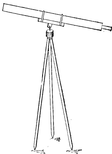
Рис. 68. Общий вид трубы на штативе
