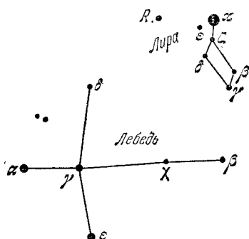
Рис. 17. Созвездия Лиры и Лебеда
