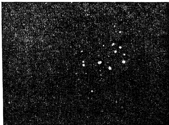
Рис. 30. Рассеянное звездное скопление Плеяды
