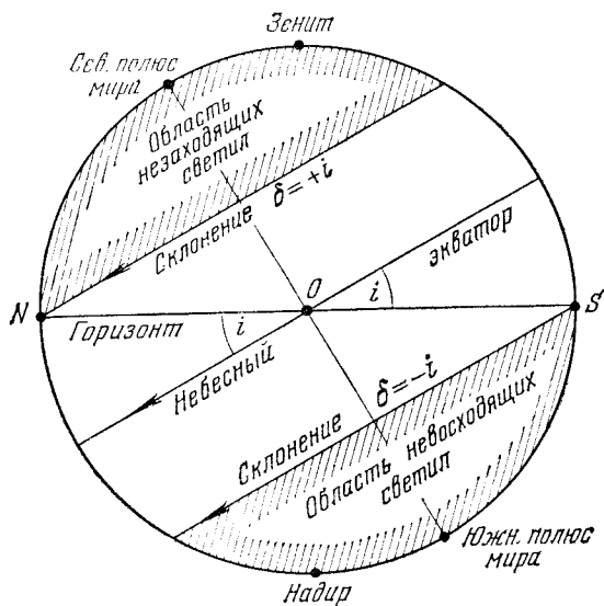
Рис. 25. Незаходящие светила ( \delta \geq +i ) и невосходящие светила ( \delta < -i ); i = 90^\circ - \varphi
