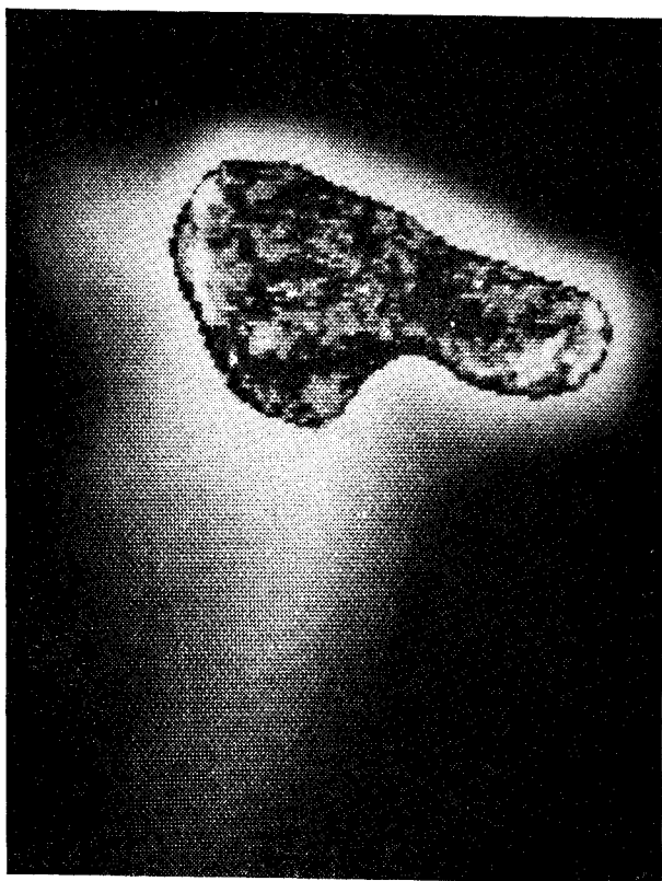
Рис. 61. Ядро кометы Галлея (фото «Веги-2»)
