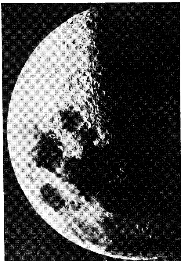
Рис. 55. Вид Луны в телескоп вблизи ее фазы первой четверти
