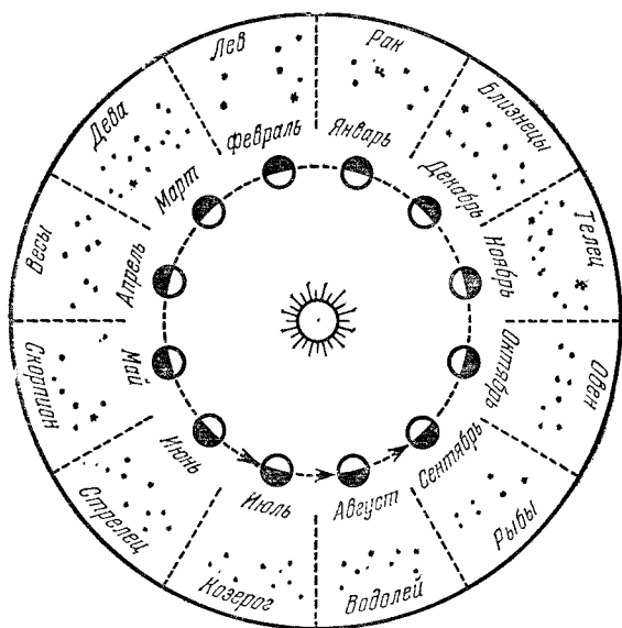
Рис. 11. Обращение Земли (в направлении стрелок) и видимое годовое движение Солнца
