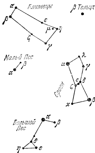
Рис. 21. Окрестности созвездия Ориона
