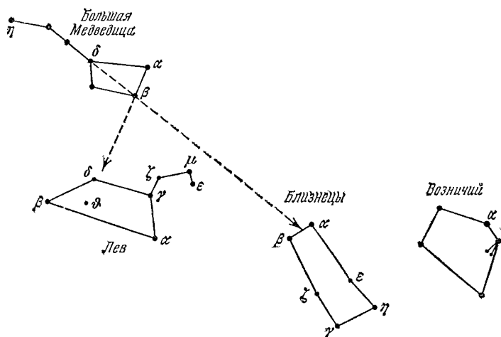
Рис. 14. Ориентировка по созвездию Большой Медведицы
