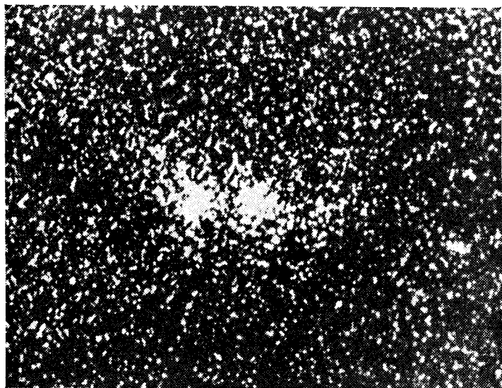
Рис. 31. Двойное рассеянное звездное скопление \eta и \chi Персея
