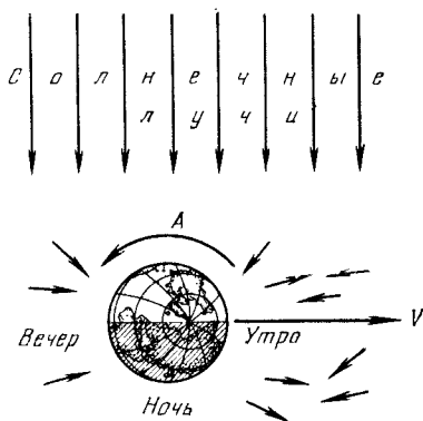
Рис. 62. Встречные и догоняющие метеоры. Стрелки: А — направление вращения Земли; V — направление скорости Земли; мелкие — направления полета метеорных частиц
