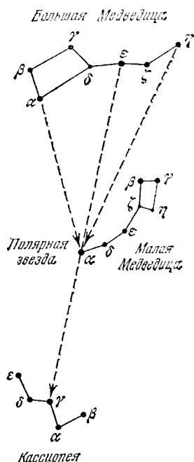
Рис. 12. Ориентировка по созвездию Большой Медведицы
