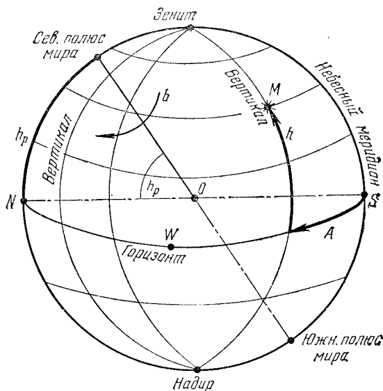
Рис. 23. Небесные горизонтальные координаты: h — высота и A — азимут светила M ; O — наблюдатель. Высота полюса мира h_p = \varphi ; S — точка юга; W — точка запада; N — точка севера; b — направление суточного вращения неба
