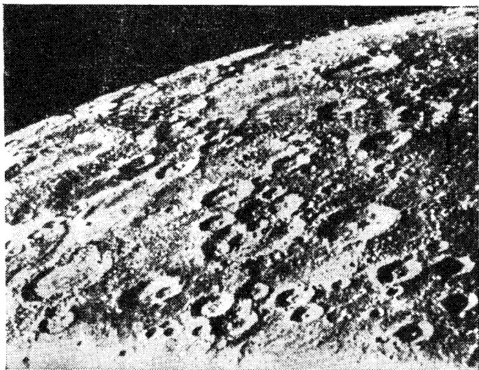
Рис. 43. Кратеры на поверхности Меркурия (фото «Маринера-10»)
