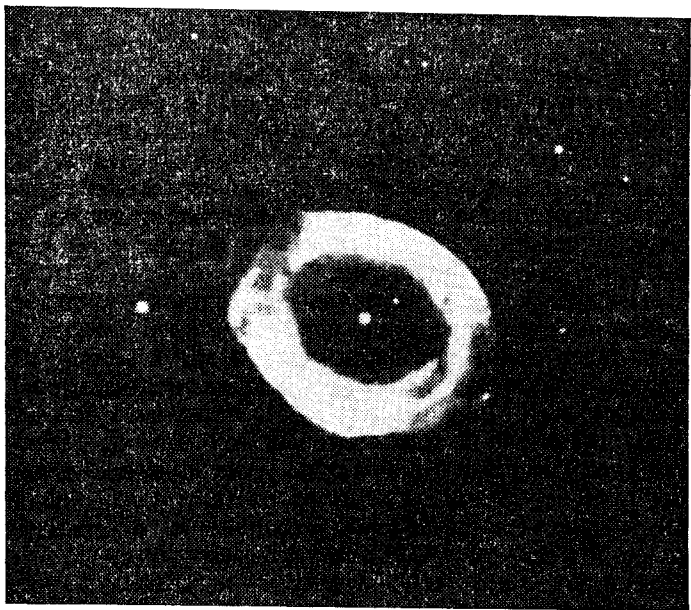
Рис. 38. Планетарная туманность «Кольцо» в созвездии Лиры
