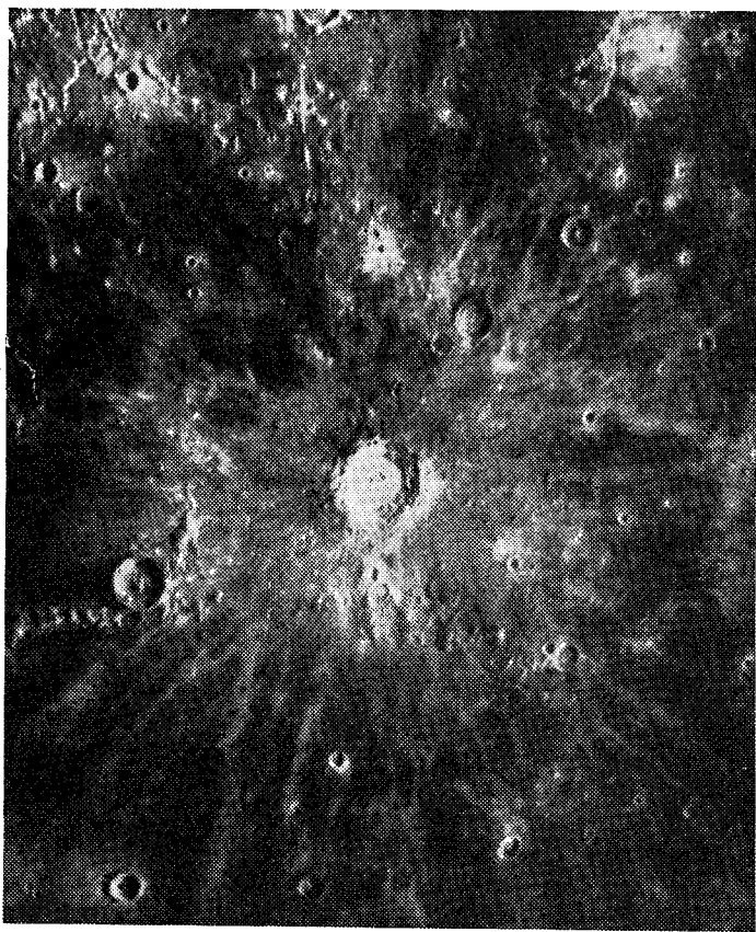
Рис. 57. Океан Бурь и кратер Коперник
