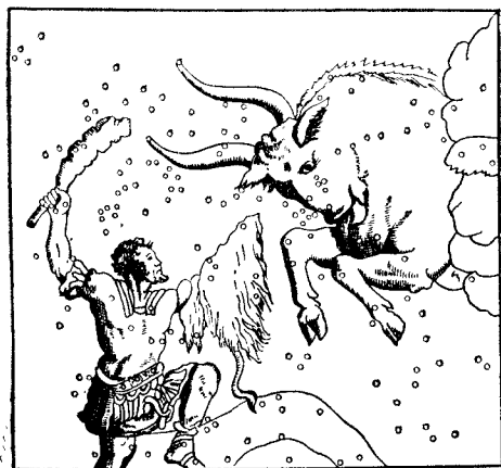
Рис. 7. Созвездия Ориона и Тельца в представлении древних греков
