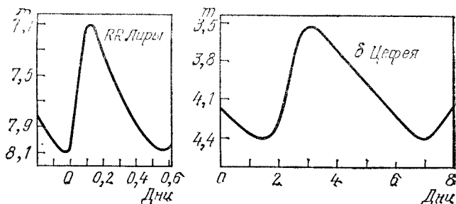
Рис. 36. Кривые блеска физических переменных звезд RR Лирь и \delta Цефея
