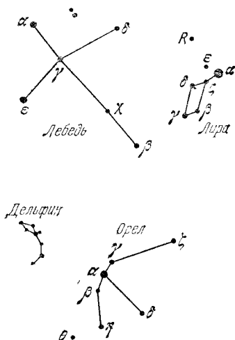
Рис. 18. Окрестности созвездия Орла
