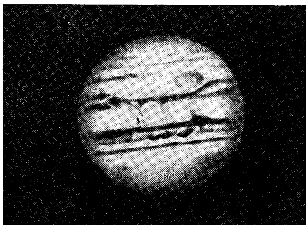
Рис. 50. Планета Юпитер
