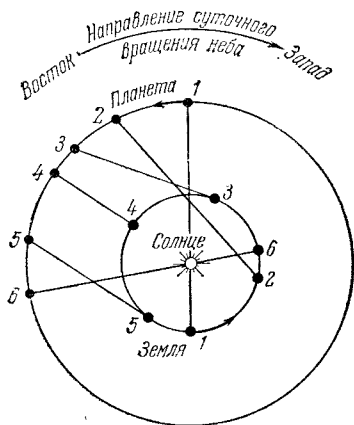
Рис. 42. Конфигурации верхних планет
