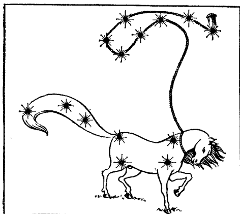
Рис. 4. Созвездия Большой и Малой Медведицы, объединенные в созвездие Коня
