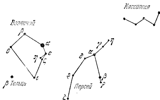
Рис. 13. Созвездия Кассиопея, Персея и Возничего
