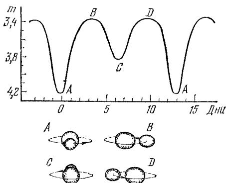
Рис. 35. Затменная переменная звезда \beta Лиры (Шелиак) и кривая ее блеска. Буквами обозначены положения звезды-спутника и соответствующие им участки кривой блеска
