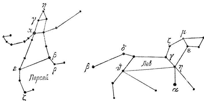
Рис. 15. Контур созвездий Персея и Льва по Г. Рею
