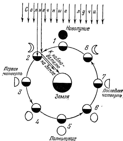
Рис. 53. Смена лунных фаз
