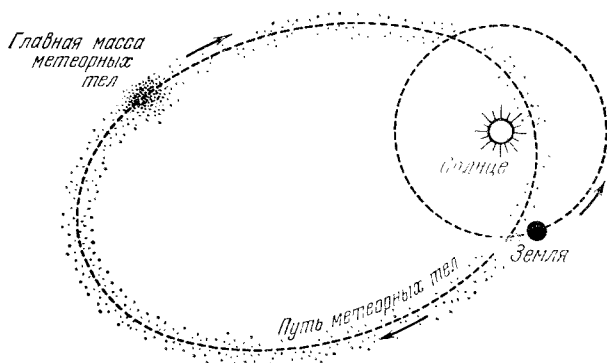
Рис. 63. Встреча Земли с метеорным потоком
