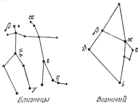
Рис. 16. Контур созвездий Близнецов и Возничего по Г. Рею
