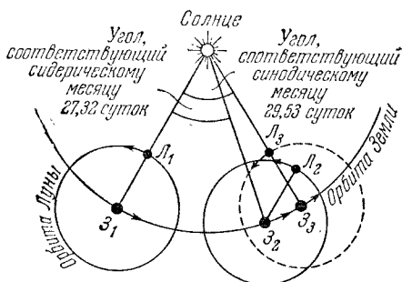
Рис. 54. Сидерический и синодический месяцы
